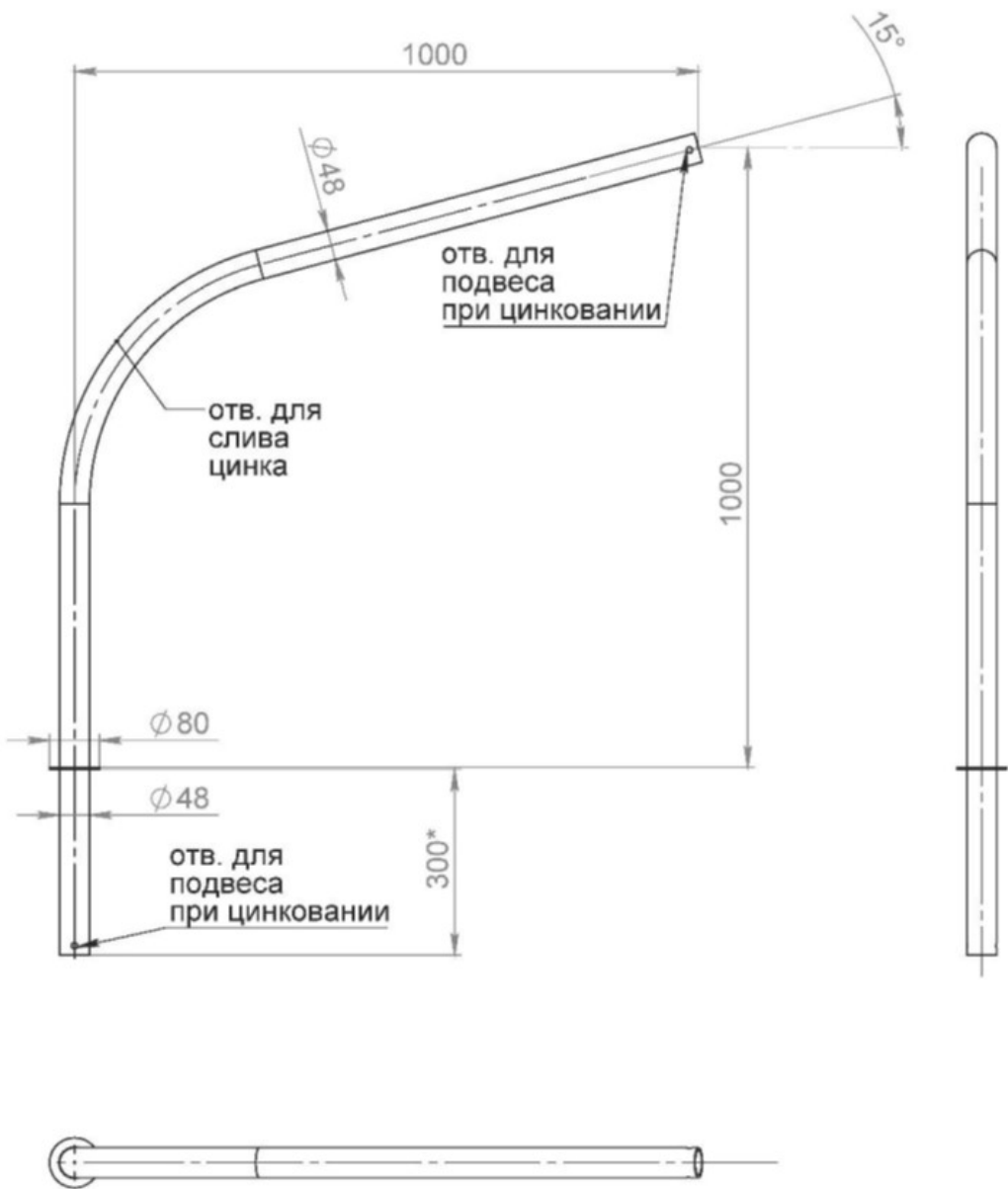
Рис.1 - Габаритные и присоединительные размеры
